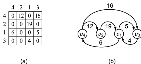
図 1 LOP のある解の行列表現 (a) とグラフ表現 (b)
